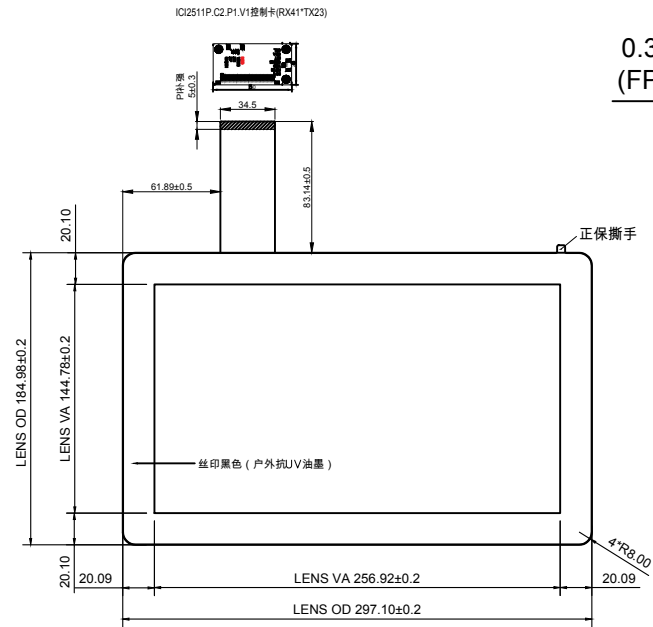
正视图
